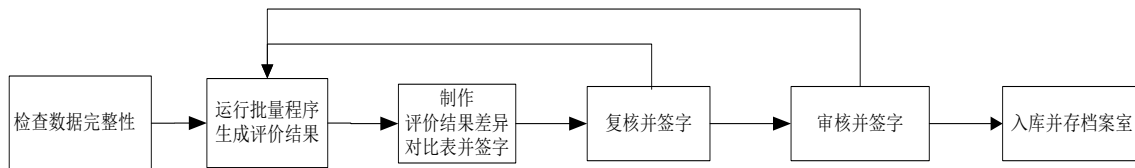
图6-11：业务流程图
