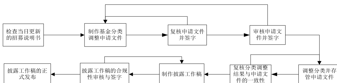
图6-8：业务流程图
