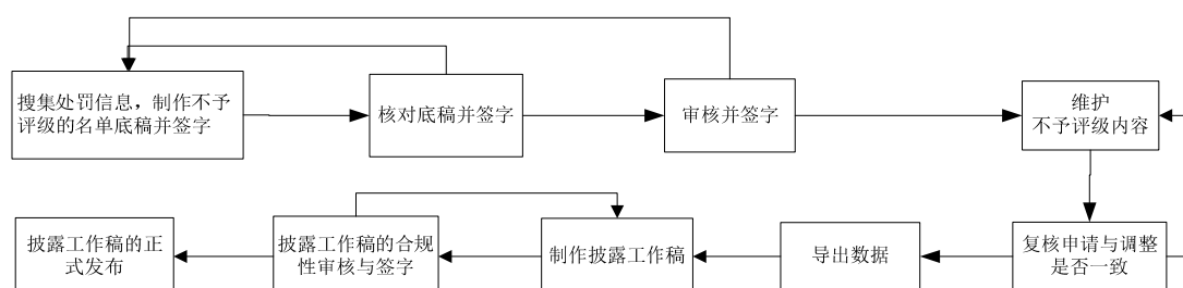
图6-9：业务流程图
