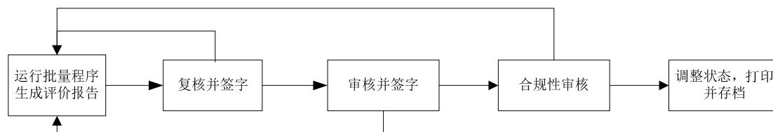
图6-12：业务流程图
