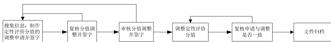
图6-10：业务流程图
