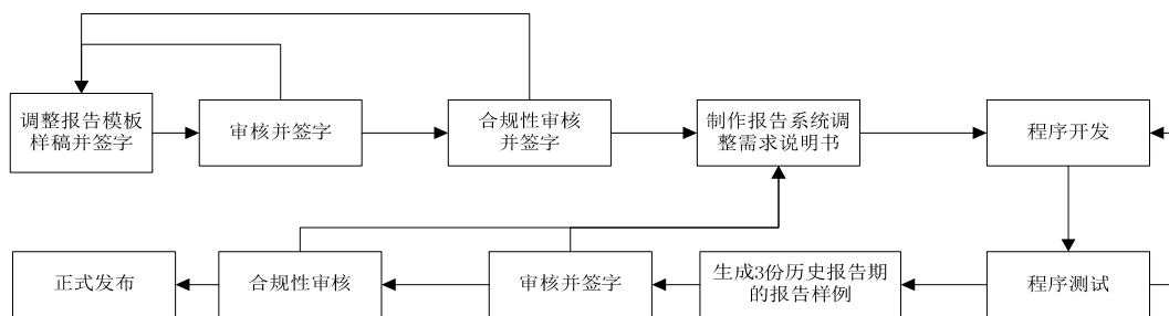
图6-14：业务流程图
