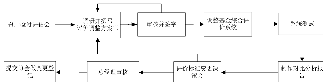
图6-15：业务流程图
