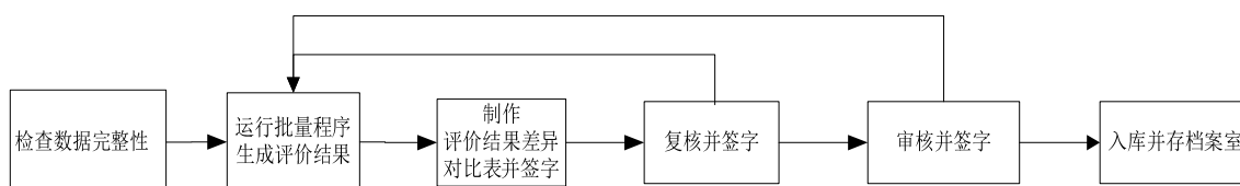
图6-11：业务流程图
