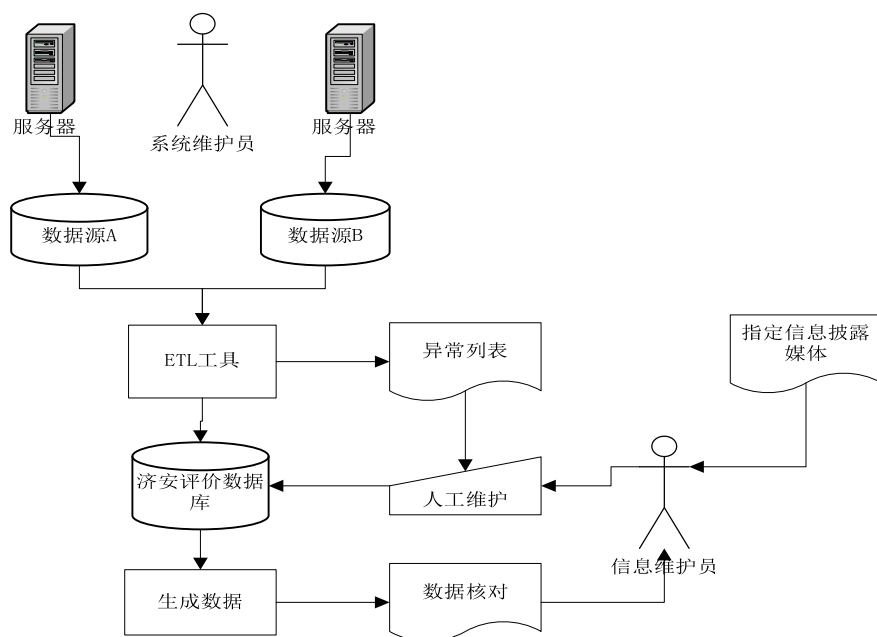
图6-7：业务流程图
